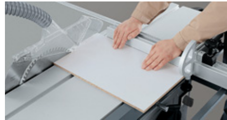
Das Reststück am Winkelanschlag auf Breitenmaß schneiden.
