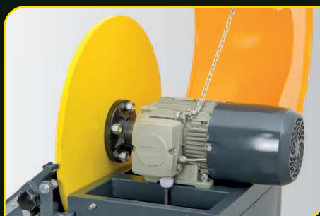
Quick disc change with self-brake Schneller Tellerwechsel mit automatischer Bremse
