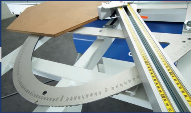
Gehrungs- und Längenausgleich SUPER-GEHRFIX I mit autom. Längenausgleich • mitre and crosscut fence SUPER-GEHRFIX I With automatic compensation of the measure • Tope de inglete y longitudinal SUPER-GEHRFIX I con compensación automática de la medida
