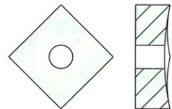
36x36x20
