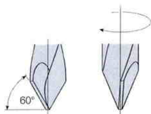
60° gennemboringsspids
